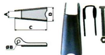
TRAVA PARA GANCHOS
