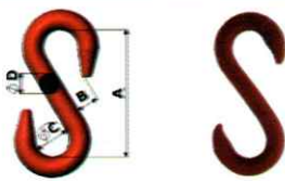
GANCHO TIPO "S" (GS)
