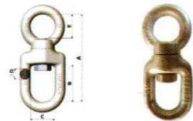
TORNEL GIRATÓRIO TIPO "PESCA" (TGP)
