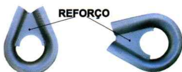
SAPATILHA P/ CABO DE AÇO (PESADA) NBR 11900/1 (SP)
