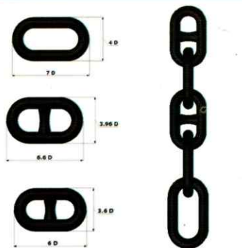
CORRENTE DE AMARRA (CRA)
