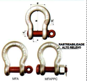
MANILHA CURVA ALLOY (MFA)
