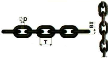
CORRENTES DE ELOS Conforme Norma EN 818-2 - GRAU 8
