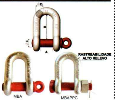
MANILHA RETA ALLOY (MBA)
