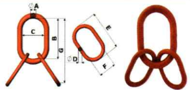
ANEL DE SUSTENTAÇÃO MASTER (ASM)
