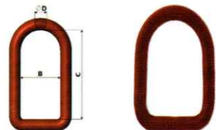
ALÇA PARA FITA (AF)
