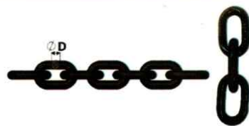
CORRENTE PARA FUNDEIO DE BÓIA DE SINALIZAÇÃO (CRFB)
